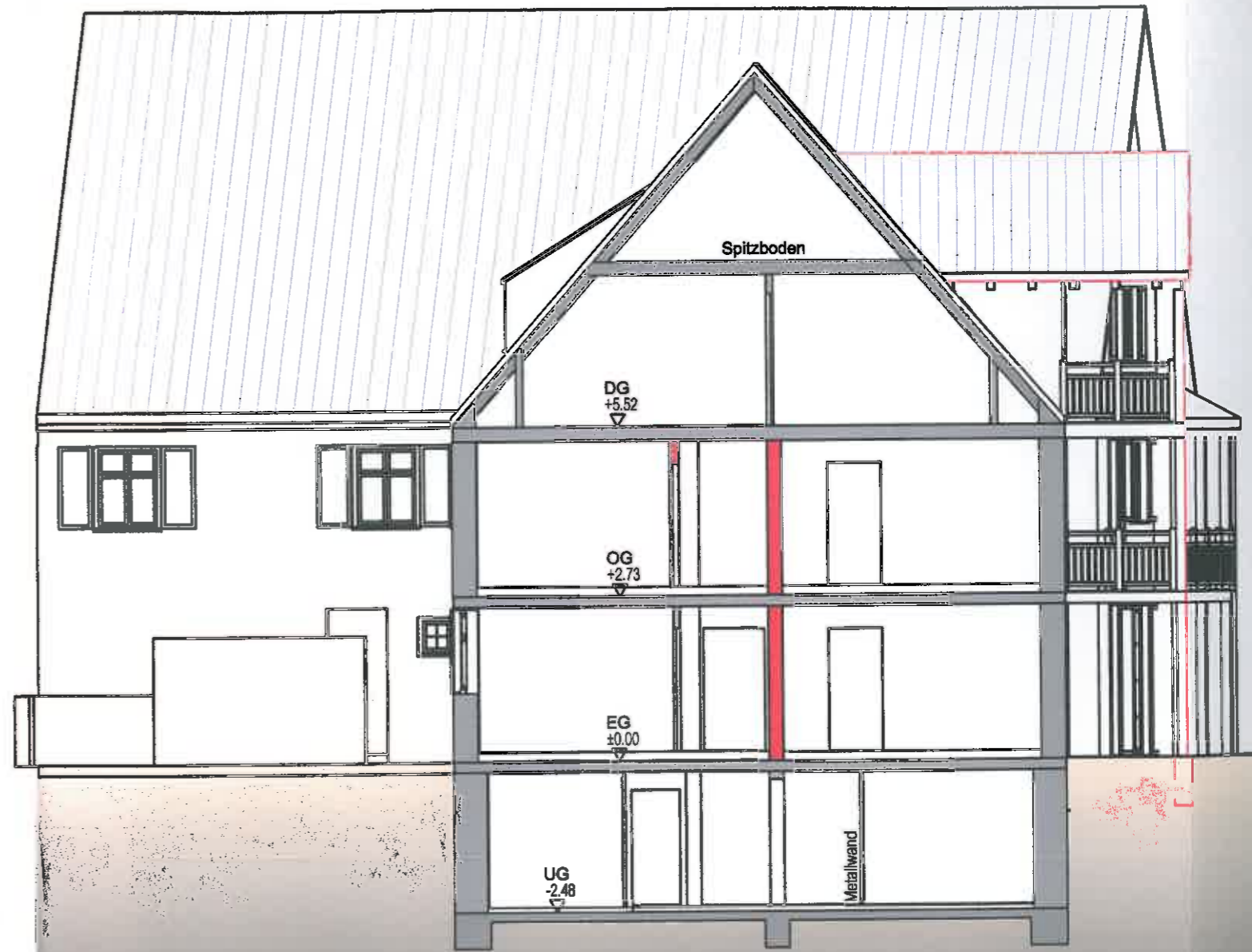
Schnitt B-B
